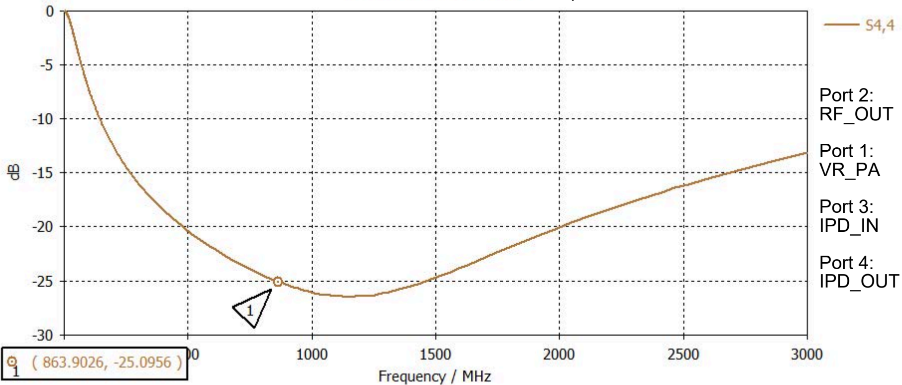
S-Parameters [Magnitude] S44 parameters for LoRa
