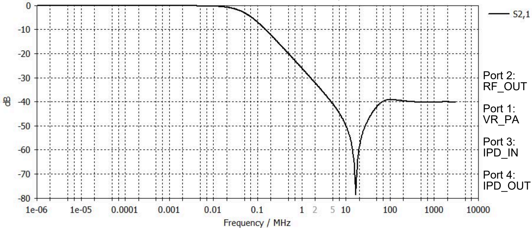
S-Parameters [Magnitude] S21 parameters for LoRa
